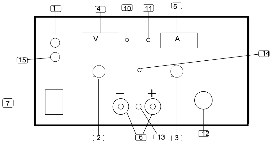
Лицевая панель GECC-1500
